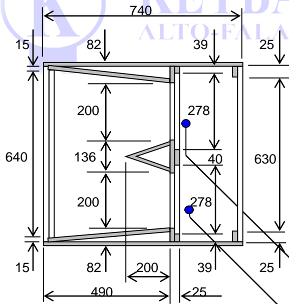
CORTE - BB
